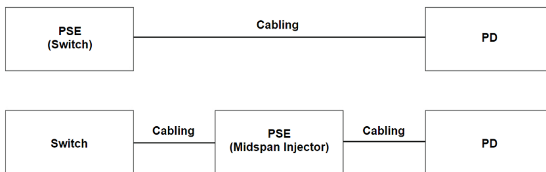
Рисунок 1. Схема организации PoE с обозначениями
